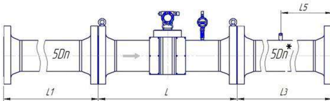
Рисунок Д.2 – Монтаж реверсивного расходомера класса точности Г (2,0 % - 1,0 %) для исполнения корпуса VR и CR с типом присоединительных фланцев по ГОСТ 33259
