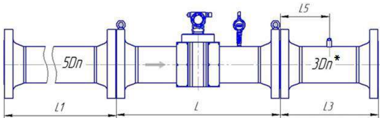
Рисунок Д.1 – Монтаж расходомера класса точности Г (2,0 % - 1,0 %) для исполнения корпуса V и С с типом присоединительных фланцев по ГОСТ 33259
