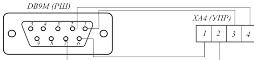
Рисунок Г.3 – Схема подключений РШ и УПР (вид контактов со стороны пайки для кабелей на рис.Г.1 и Г.2)
