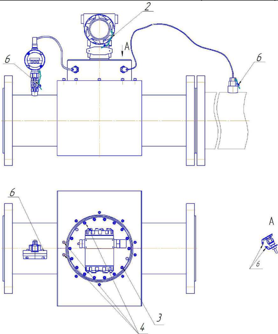
Рисунок Е.2 – Схема пломбирования расходомера Turbo Flow UFG-F исполнение корпуса V, VR
