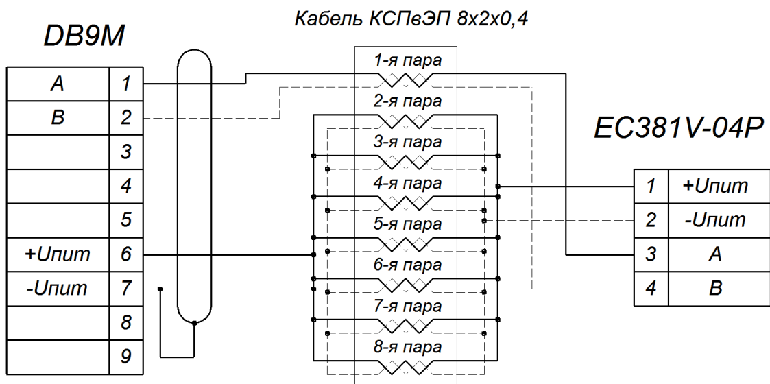
Рисунок Г.2 – Схема распайки кабеля КСПвЭП 8×2×0,4
