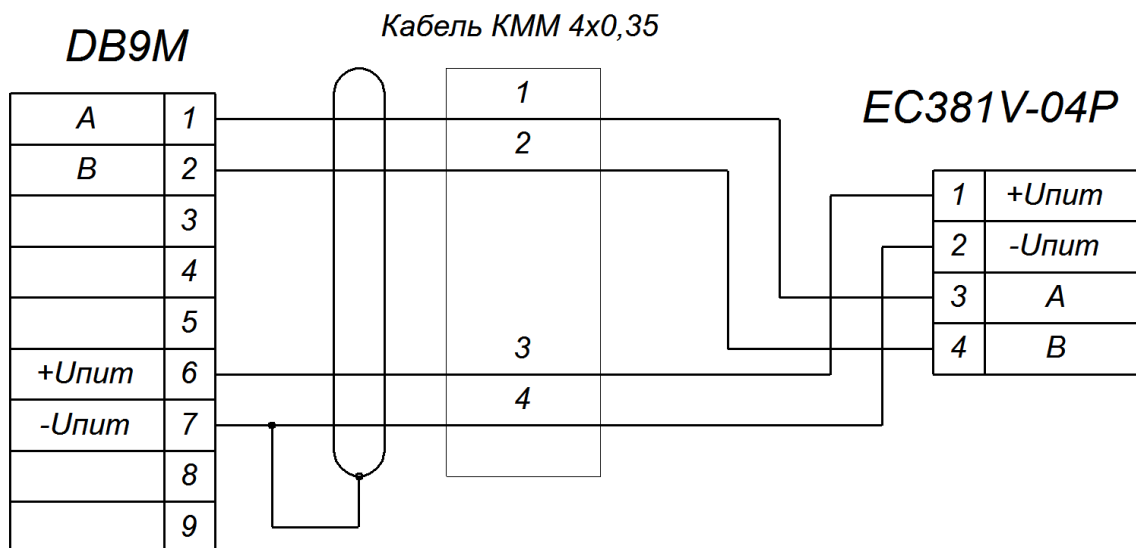
Рисунок Г.1.1 – Схема распайки кабеля КММ 4×0,35
