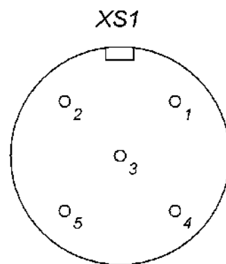
Рисунок Г.5 – Разъемы для подключения термосопротивления (вид со стороны пайки кабельного разъема)
