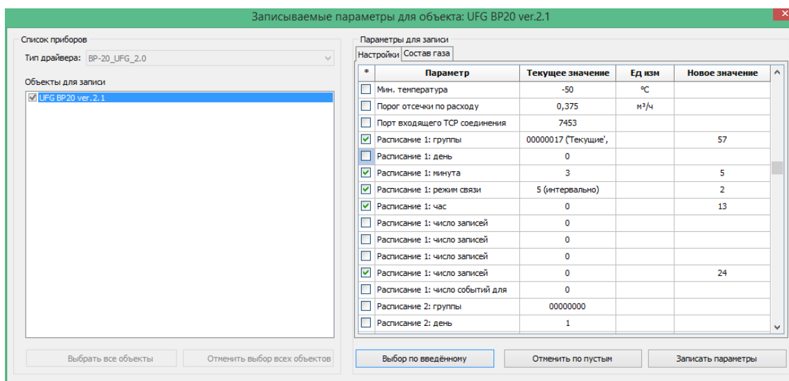
Рисунок М.36. Окно настройки параметров на запись
