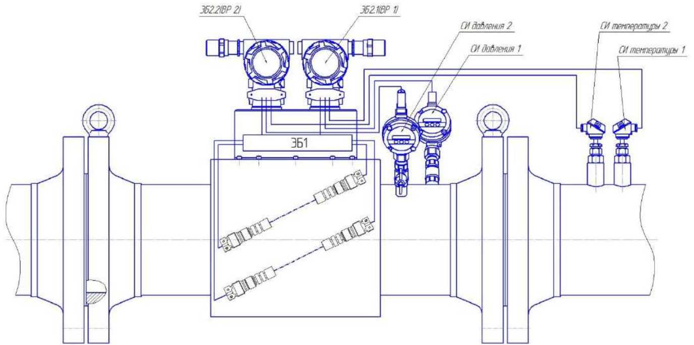
Рисунок Б.6 – Дублирование вычислительных средств и СИ температуры и давления (исполнение С1ТР, С2ТР)
