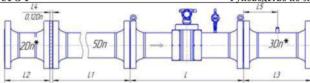
Рисунок Д.12 – Монтаж расходомера со струевыпрямителем укороченной длины со вставкой 2 Dn классов точности А (0,5 %-0,3 %) и Б (0,5 %-0,5 %) для исполнения корпуса V по стандарту ASME B16.5-2003
