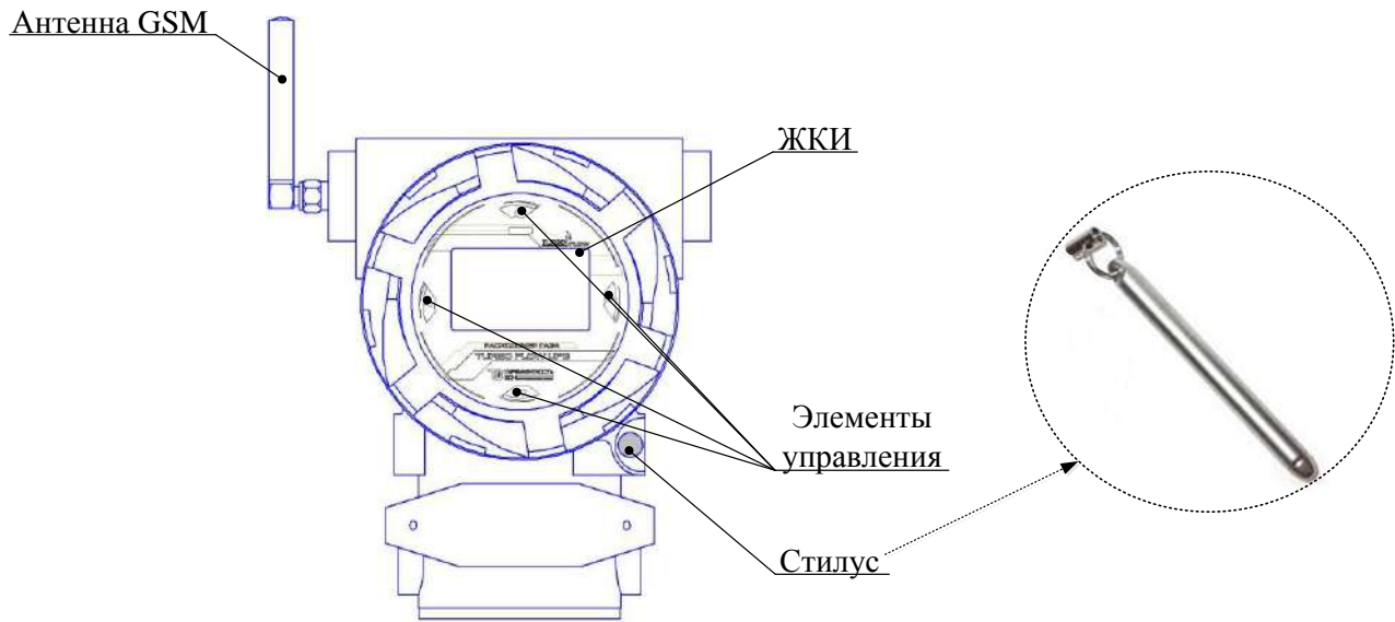
Рисунок Б.13 – Внешний вид электронного блока
