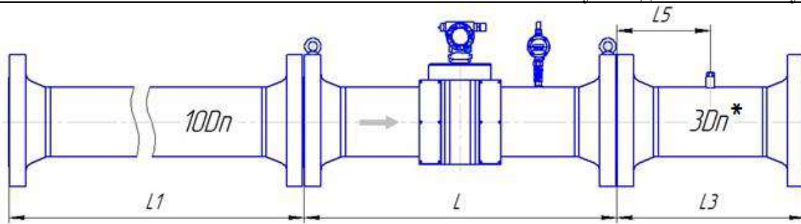
Рисунок Д.4 – Монтаж расходомера класса точности В (1,0 % - 1,0 %) для исполнения корпуса V и С с типом присоединительных фланцев по ГОСТ 33259
