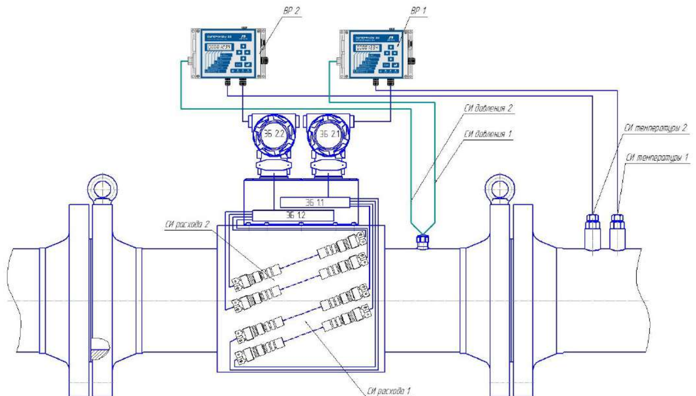
Рисунок Б.12 – Дублирование средств измерения расхода, вычислительных средств и СИ температуры и давления (исполнение С4)
