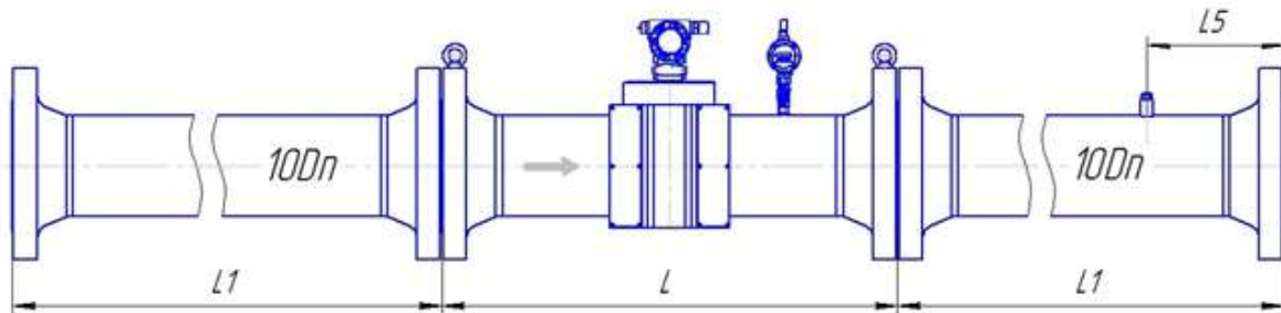
Рисунок Д.9 – Монтаж реверсивного расходомера класса точности В (1,0 % - 1,0 %) для исполнения корпуса VR и CR с типом присоединительных фланцев по ГОСТ 33259
