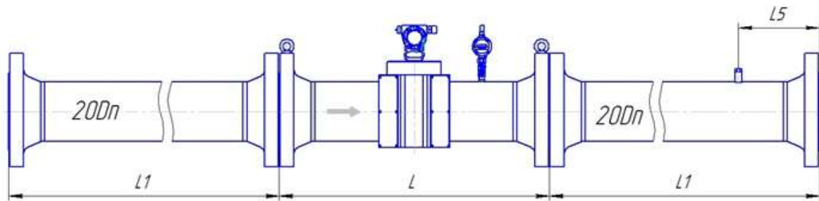
Рисунок Д.16 – Монтаж реверсивного расходомера классов точности А (0,5 % - 0,3 %) и Б (0,5 % - 0,5 %) для исполнения корпуса VR по стандарту ASME B16.5-2003
