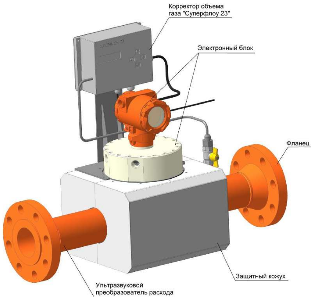
Рисунок Б.8 – Расходомер - счетчик газа ультразвуковой исполнение корпуса V, VR с корректором «Суперфлюу 23» (исполнение С4)
