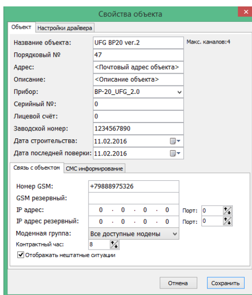
Рисунок М.27 Вкладка общих свойств объекта
