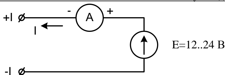
Рисунок 4.6 Схема подключения приборов для проверки токового выхода
