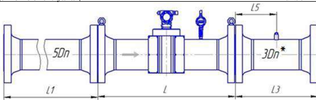
Рисунок Д.15 – Монтаж расходомера класса точности Г (2,0 % - 1,0 %) для исполнения корпуса V по стандарту ASME B16.5-2003
