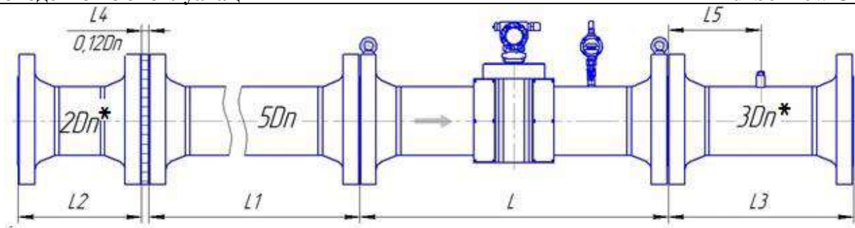
Рисунок Д.5 – Монтаж расходомера со струевыпрямителем со вставкой 2Dn класса точности В (1,0 % - 1,0 %) для исполнения корпуса V и С с типом присоединительных фланцев по ГОСТ 33259
