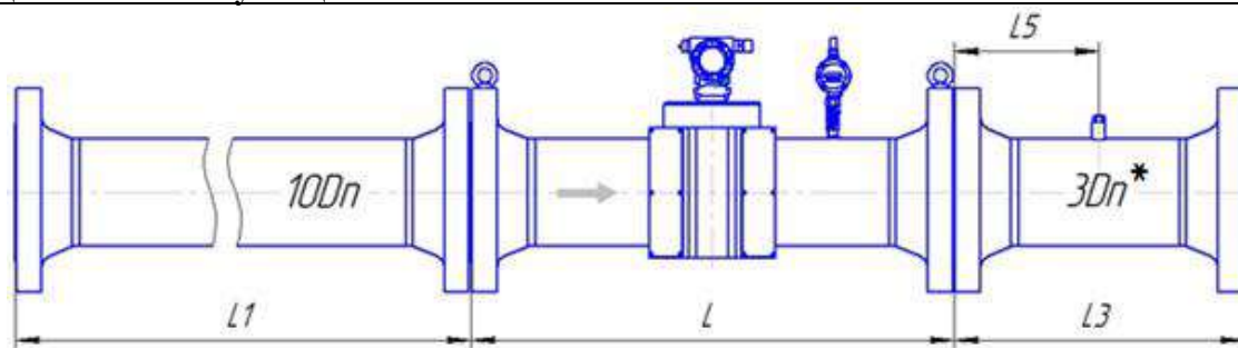
Рисунок Д.13 – Монтаж расходомера класса точности В (1,0 % - 1,0 %) для исполнения корпуса V по стандарту ASME B16.5-2003
