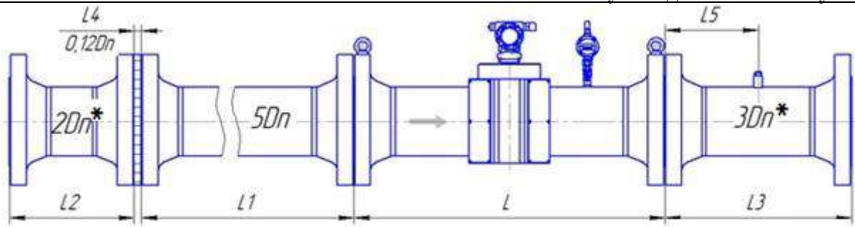
Рисунок Д.14 – Монтаж расходомера со струевыпрямителем со вставкой 2Dn класса точности В (1,0 % - 1,0 %) для исполнения корпуса V по стандарту ASME B16.5-2003
