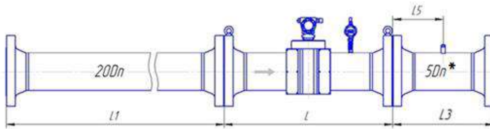
Рисунок Д.1 – Монтаж расходомера классов точности А (0,5 % - 0,3 %) и Б (0,5 % - 0,5 %) для исполнения корпуса V и С с типом присоединительных фланцев по ГОСТ 33259
