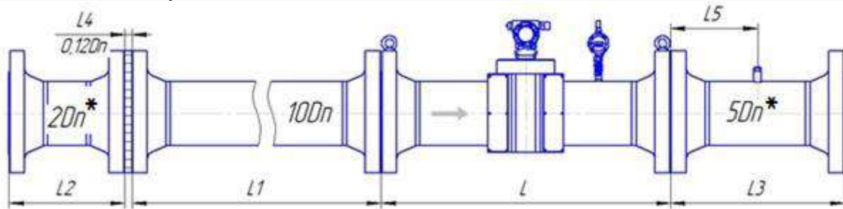
Рисунок Д.11 – Монтаж расходомера со струевыпрямителем со вставкой 2 Dn классов точности А (0,5 % - 0,3 %) и Б (0,5% - 0,5%) для исполнения корпуса V по стандарту ASME B16.5-2003
