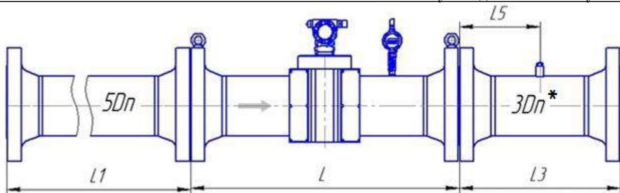
Рисунок Д.6 – Монтаж расходомера класса точности Г (2,0 % - 1,0 %) для исполнения корпуса V и С с типом присоединительных фланцев по ГОСТ 33259
