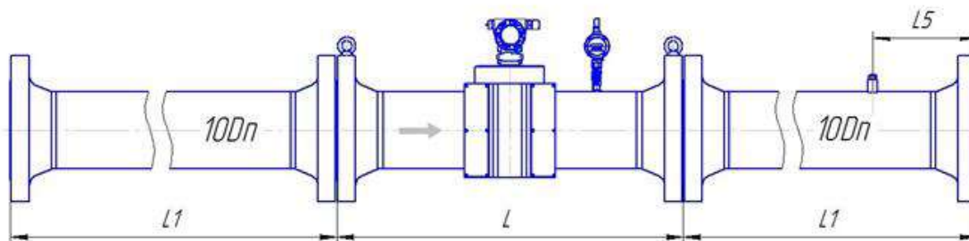
Рисунок Д.17 – Монтаж реверсивного расходомера классов точности В (1,0 % - 1,0 %) для исполнения корпуса VR по стандарту ASME B16.5-2003
