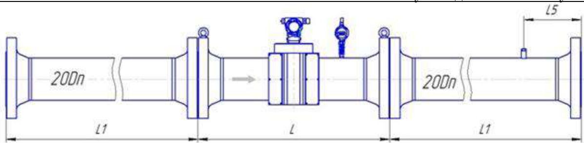
Рисунок Д.8 – Монтаж реверсивного расходомера классов точности А (0,5 % - 0,3 %) и Б (0,5 % - 0,5 %) для исполнения корпуса VR и CR с типом присоединительных фланцев по ГОСТ 33259
