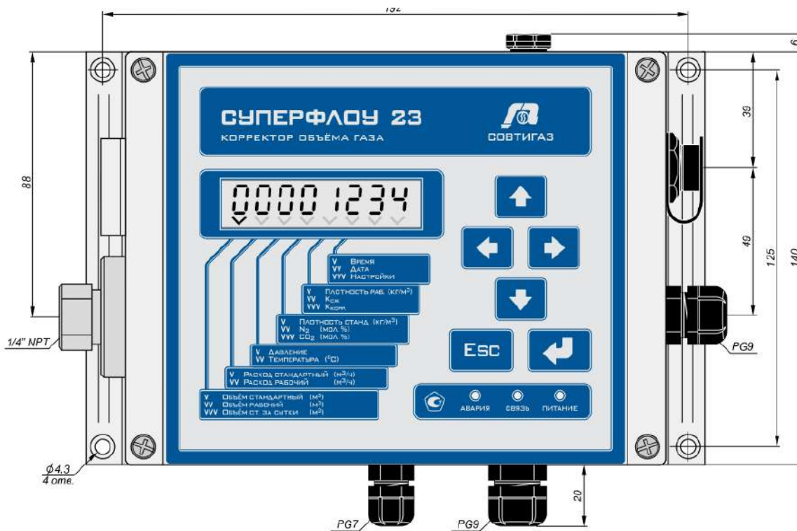
Рисунок Б.8 – Расходомер - счетчик газа ультразвуковой исполнение корпуса V, VR с корректором «Суперфлюу 23» (исполнение С4)
