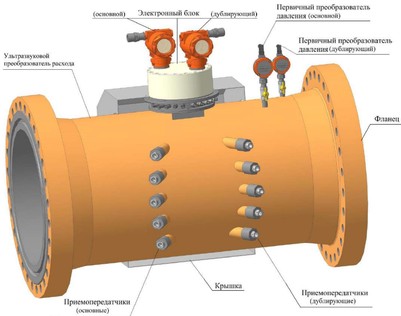
Рисунок Б.5– Расходомер - счетчик газа ультразвуковой исполнение дублирование средств измерений согласно СТО Газпром 5-37-2011
