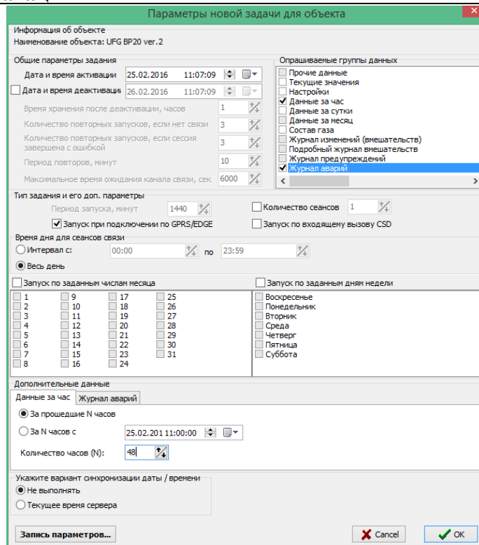
Рисунок М.35. Окно постановки автоматического задания
