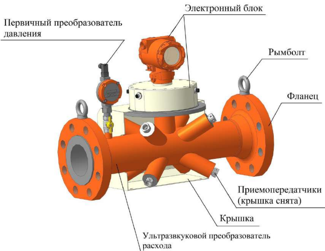
Рисунок Б.3 – Расходомер - счетчик газа ультразвуковой исполнение корпуса V, VR
