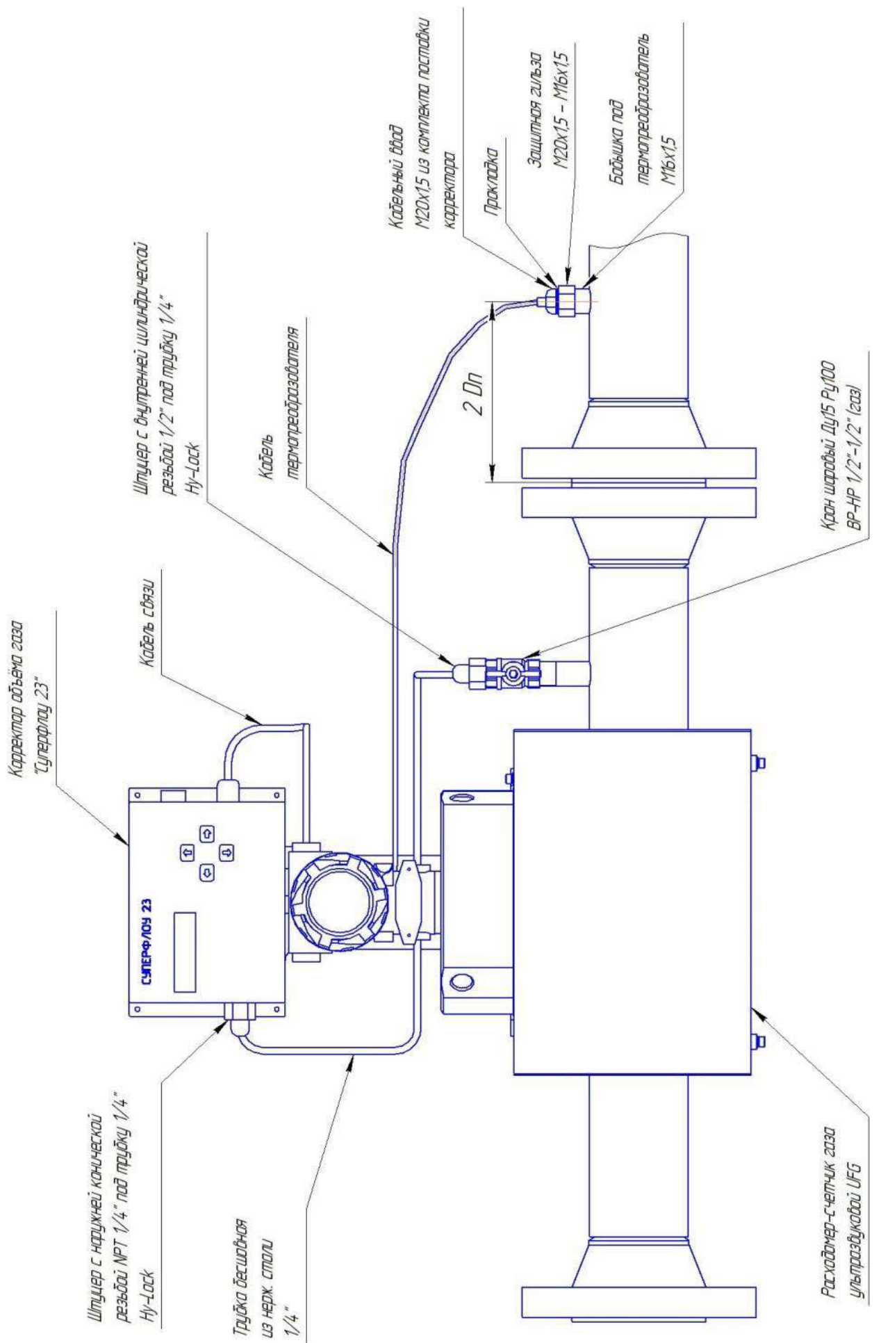
Рисунок Б.10 – Чертеж монтажный
