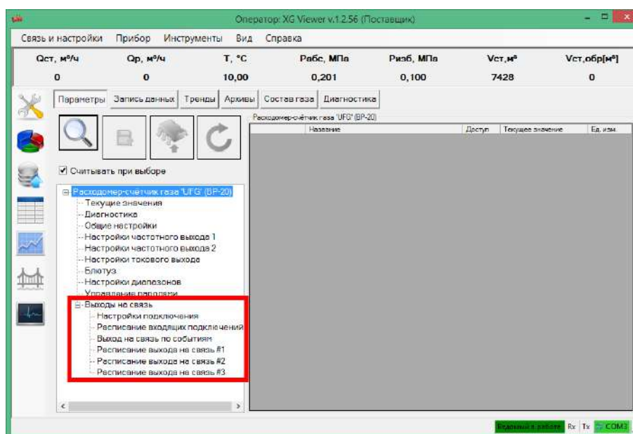
Рисунок М.8. Группа параметров "Выходы на связь" в дереве параметров ПО «XG Viewer»
