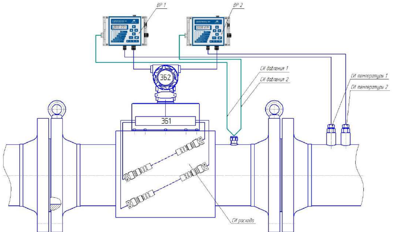
Рисунок Б.11 – Дублирование вычислительных средств и СИ температуры и давления (исполнение С4)
