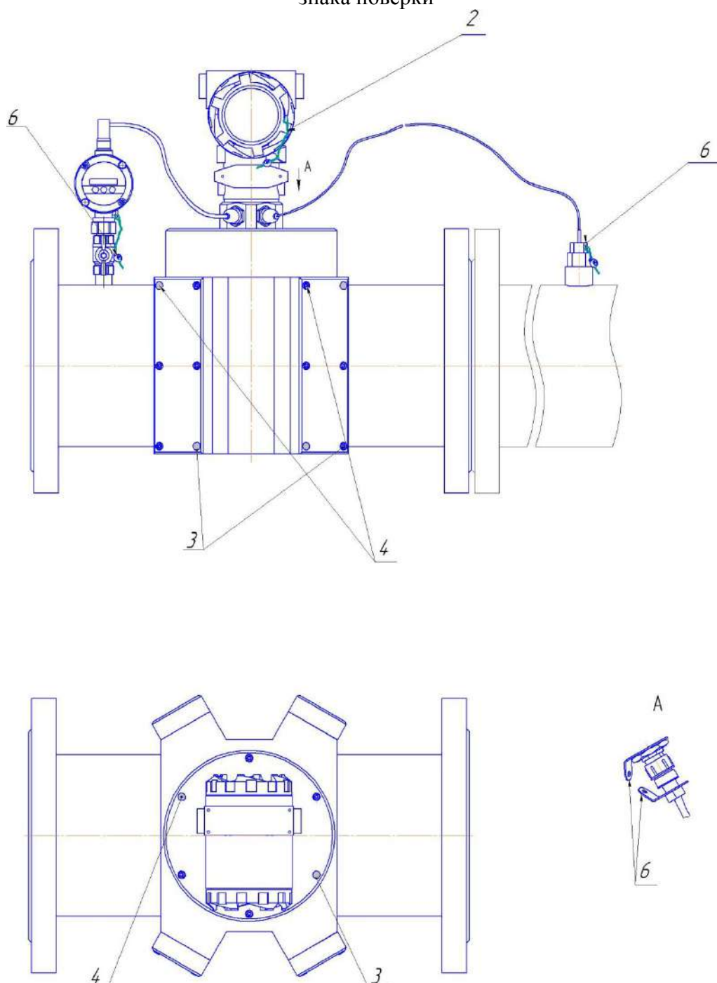
Рисунок Е.1 – Схема пломбирования расходомера Turbo Flow UFG-F исполнение корпуса D, DR
