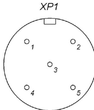
Рисунок Г.4 – Разъемы для подключения датчика давления (вид со стороны пайки кабельного разъема)
