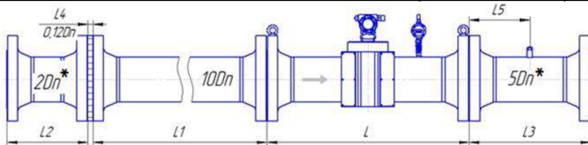
Рисунок Д.2–Монтаж расходомера со струевыпрямителем со вставкой 2Dn классов точности А (0,5% - 0,3%) и Б (0,5%-0,5%) для исполнения корпуса V и С с типом присоединительных фланцев по ГОСТ 33259
