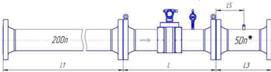
Рисунок Д.10 – Монтаж расходомера классов точности А (0,5 % - 0,3 %) и Б (0,5 % - 0,5 %) для исполнения корпуса V с типом присоединительных фланцев по стандарту ASME B16.5-2003
