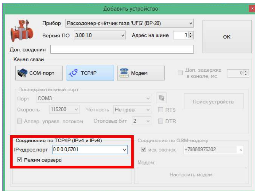
Рисунок М.5. Поле настройки параметров канала "TCP/IP"
