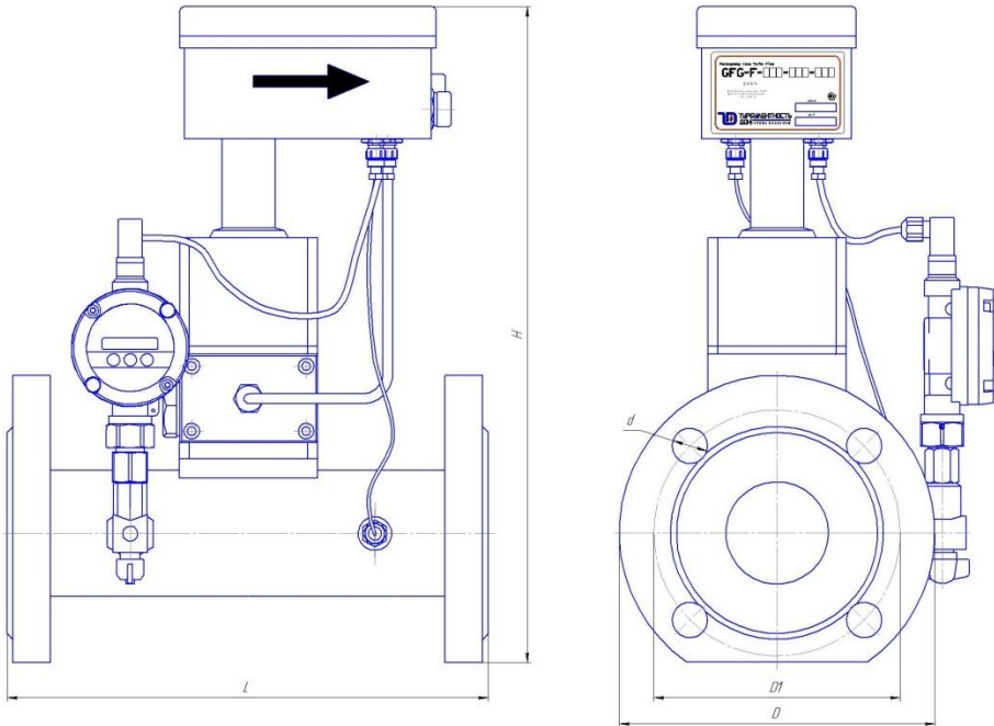
Рисунок В.1 Габаритно-присоединительные размеры ПР расходомеров исполнения GFG-F-XXX-XXX-XXX.XX
