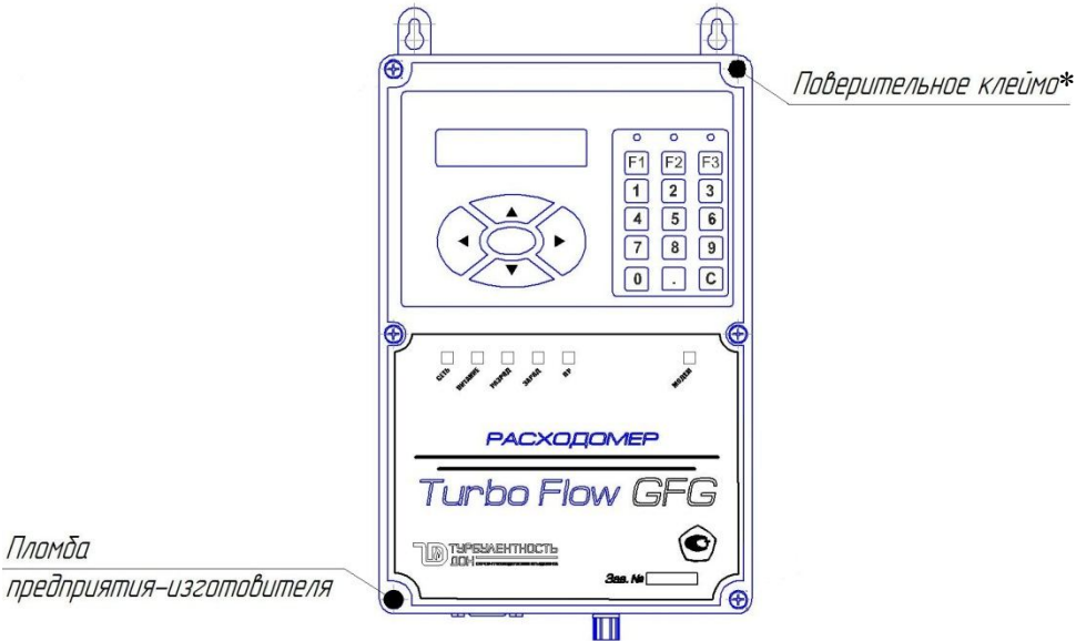
Рисунок Д.2 Пломбирование РШ
