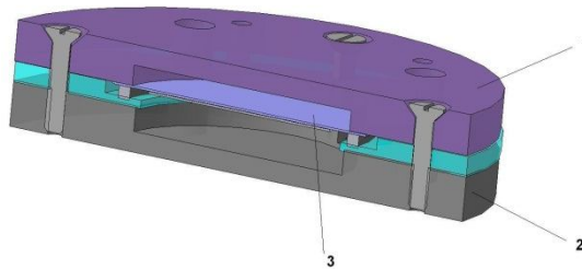
Рисунок 2 – Пьезодатчик
