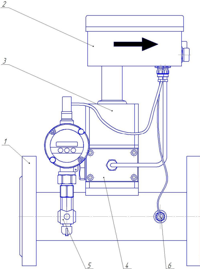
Рисунок Б.1 Общий вид ПР расходомеров исполнения GFG-F-XXX-XXX-XXX.XX
