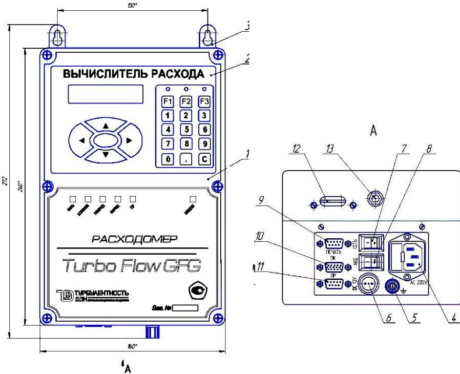
ПРИЛОЖЕНИЕ Г Рисунок Г.1 Внешний вид РШ
