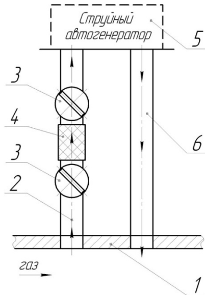
Рисунок 4 – Схема фильтра
