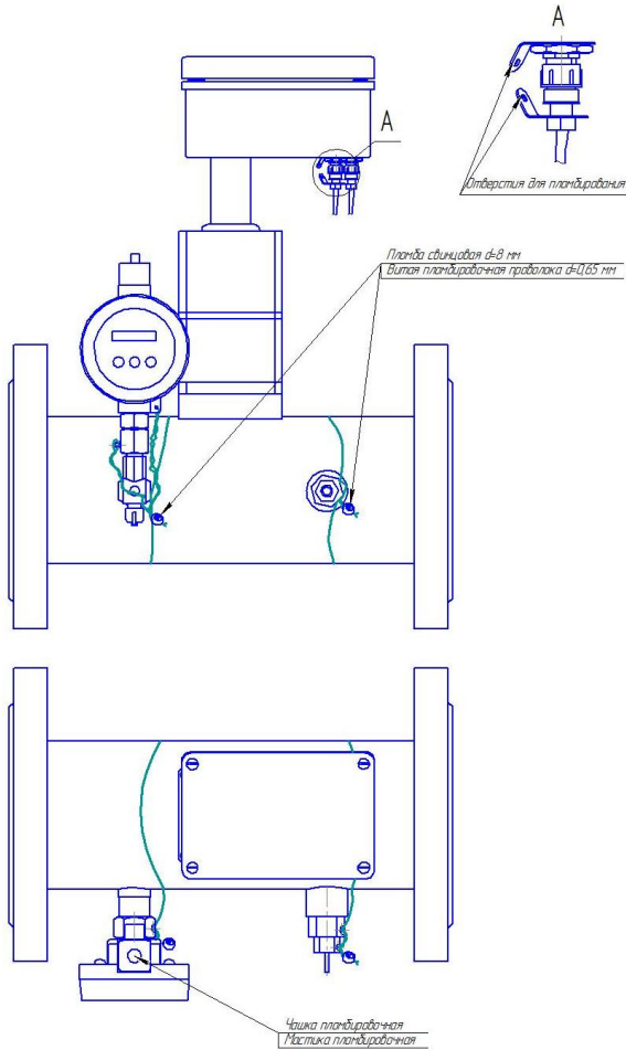
Рисунок Д.3 Пломбирование ПР
