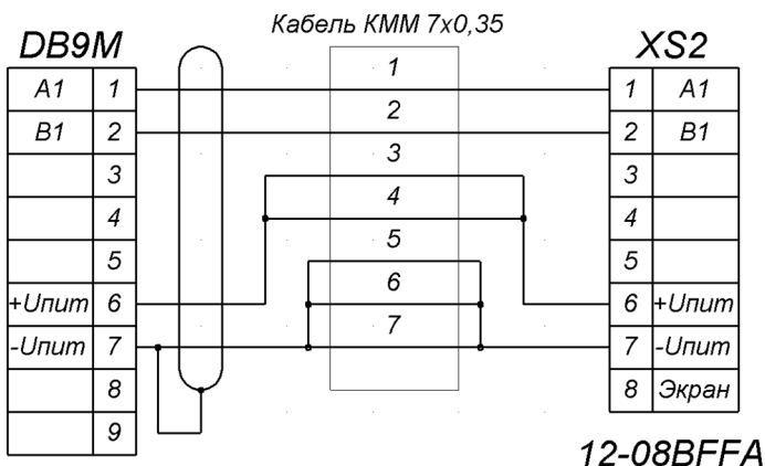
Рисунок И.1. Схема распейки кабеля КММ 7x0,35
