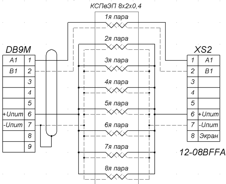
Рисунок И.2. Схема распейки кабеля КСПвЭП 8x2x0,4
