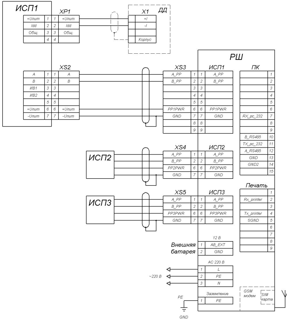
Рисунок Л.2 – Схема подключений при использовании разъемов 2РМ
