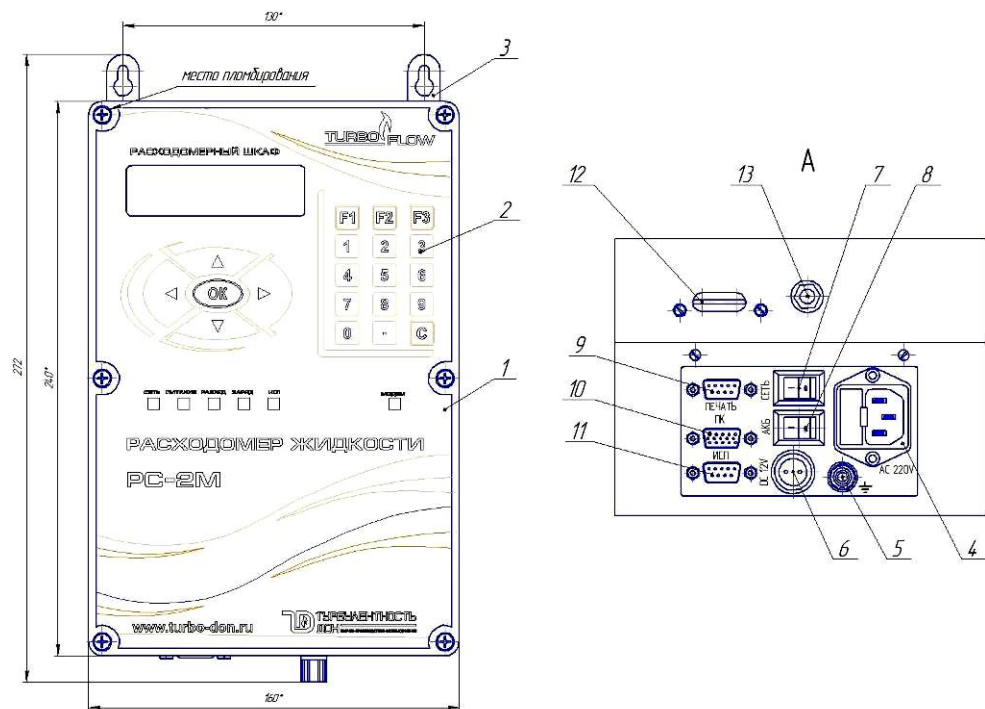
Рисунок В.1 – Внешний вид расходомерного шкафа для одноканального расходомера
