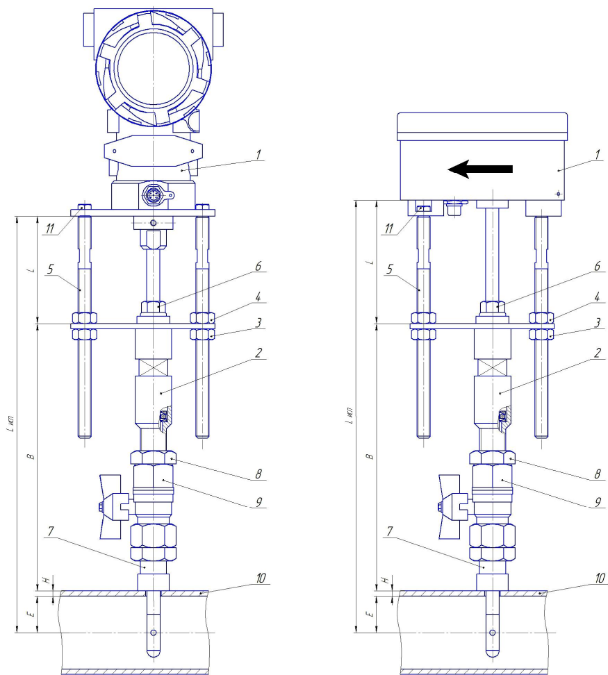
Рисунок Ж.1 – Монтаж расходомера РС-2М на стальную трубу
