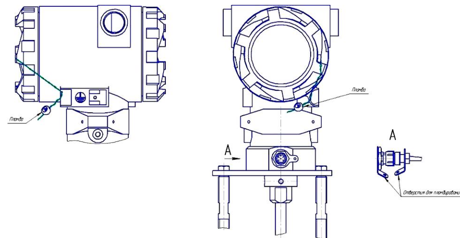
Рисунок Б.2.1 – Схема пломбирования
