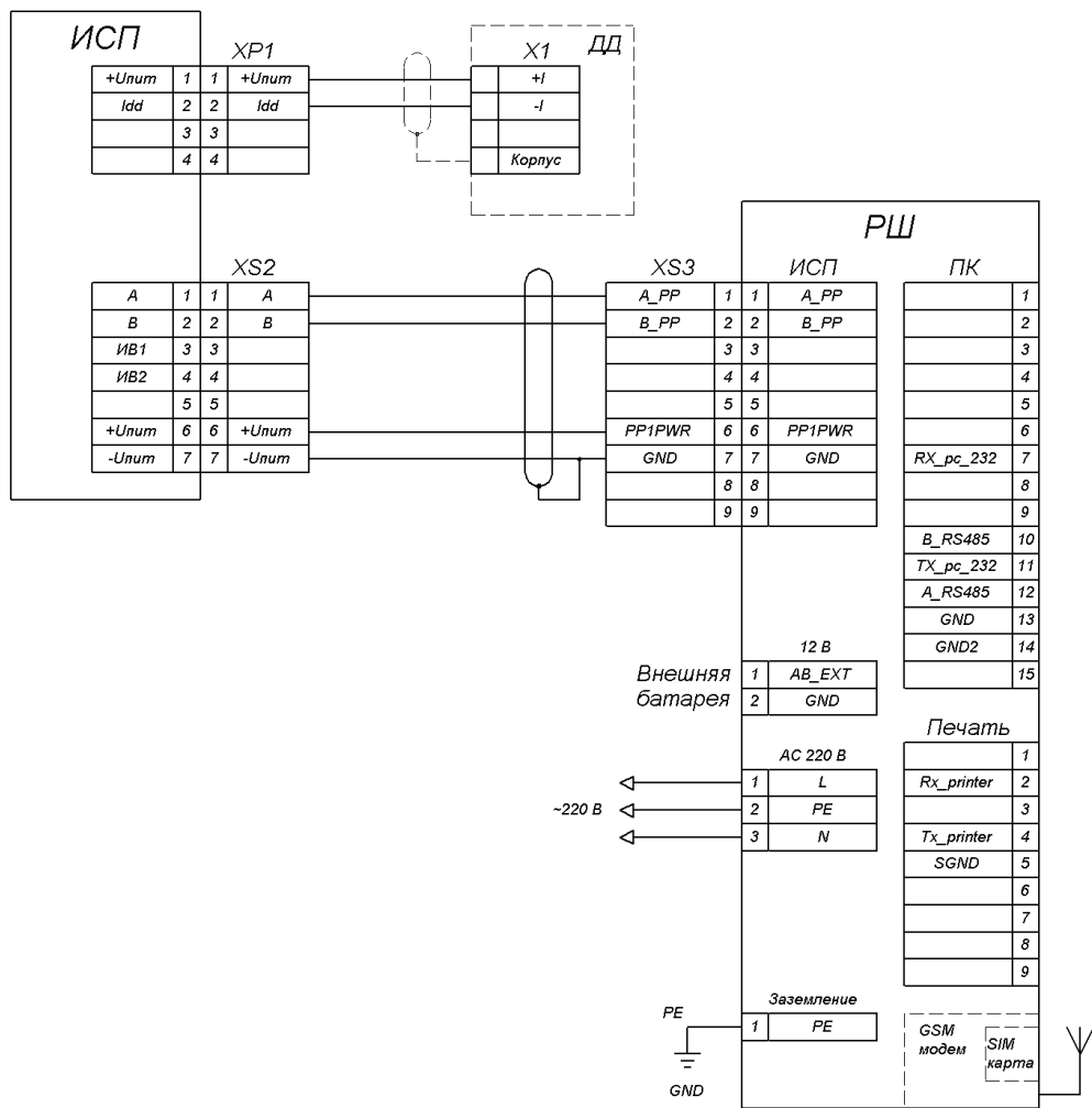
Рисунок К.2 – Схема подключений при использовании разъемов 2PM
