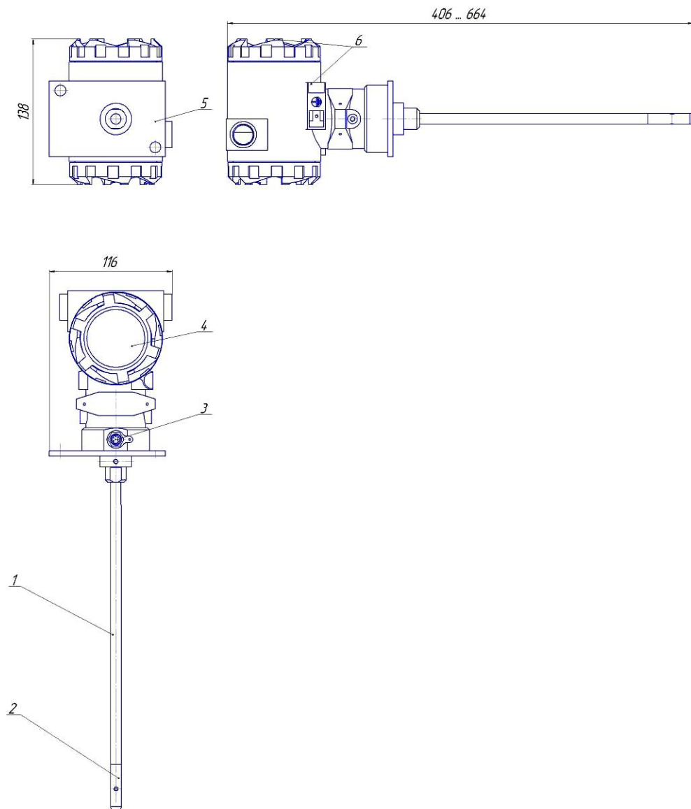
Рисунок Б.2 – Внешний вид блока ИСП с индикацией
