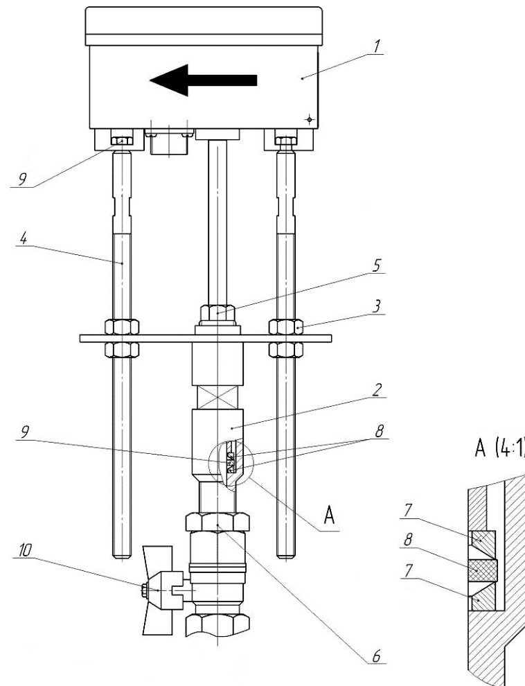
Рисунок Е.2 – Конструкция ввода на пластиковую трубу
