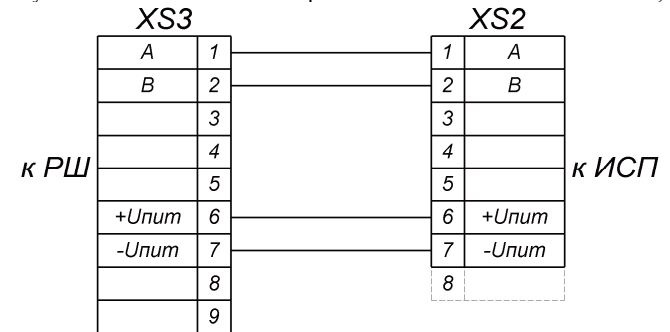
Рисунок М.3 – Проверочный системный кабель
