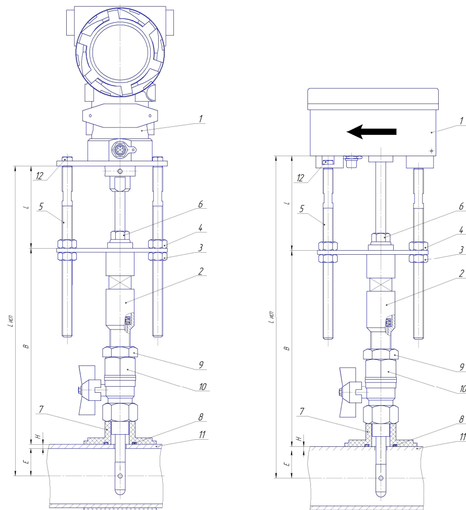
Рисунок Ж.2 – Монтаж расходомера РС-2М на пластиковую трубу
