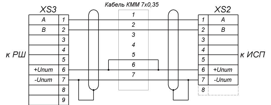
Рисунок М.1 – Схема кабеля при использовании КММ 7x0,35
