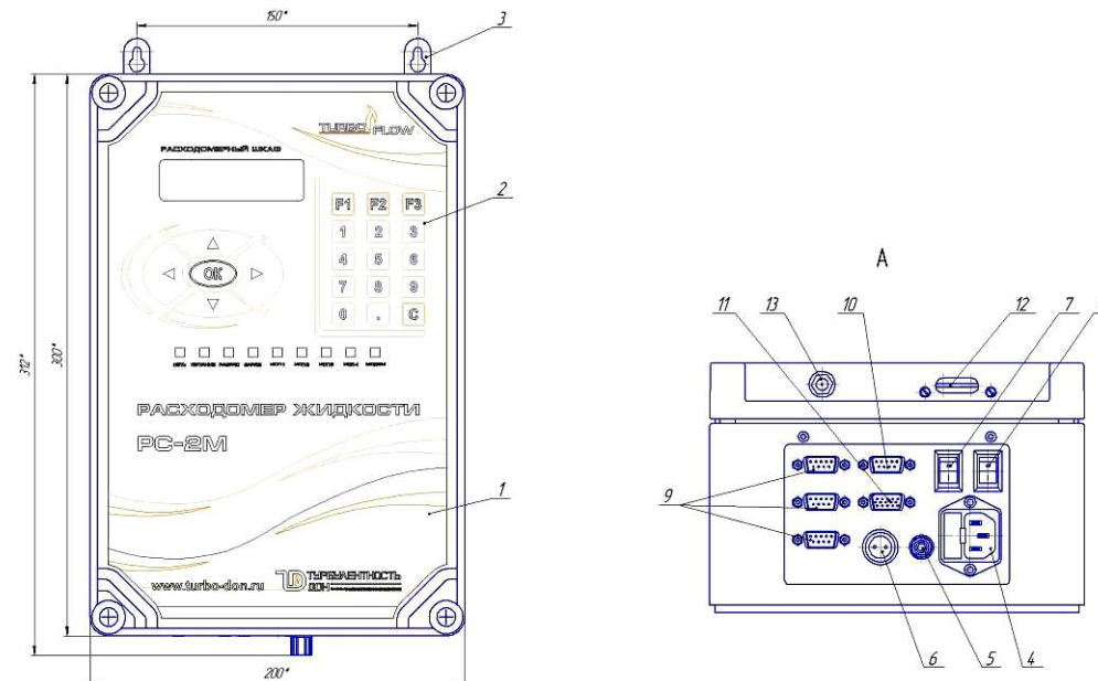
Рисунок В.2 – Внешний вид расходомерного шкафа для многоканального расходомера
