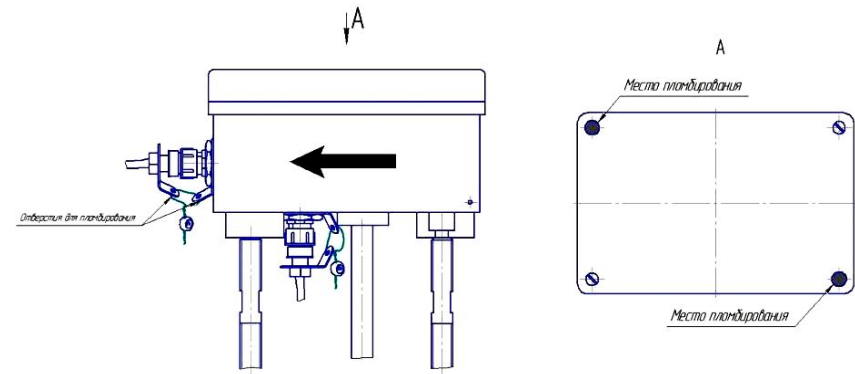
Рисунок Б.1.1 – Схема пломбирования
