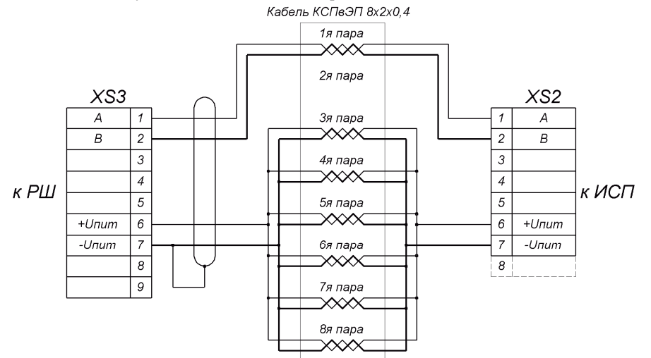
Рисунок М.2 – Схема кабеля при использовании КСПвЭП 8x2x0,4
