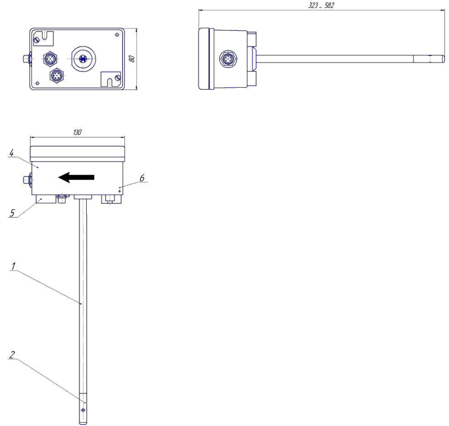
Рисунок Б.1 – Внешний вид блока ИСП (с разъемами LTW)
