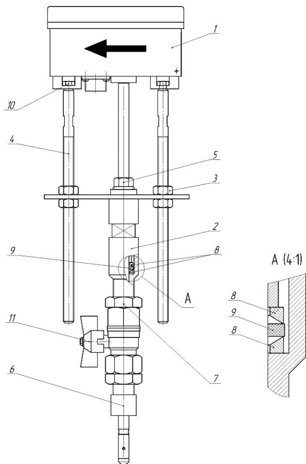
Рисунок Е.1 – Конструкция ввода на стальную трубу
